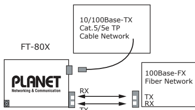
Рисунок 8: Установка FT-80x
